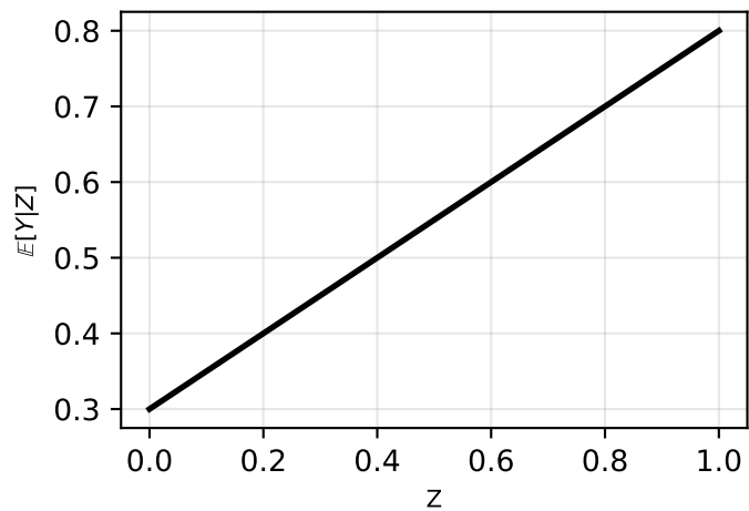
Linear
